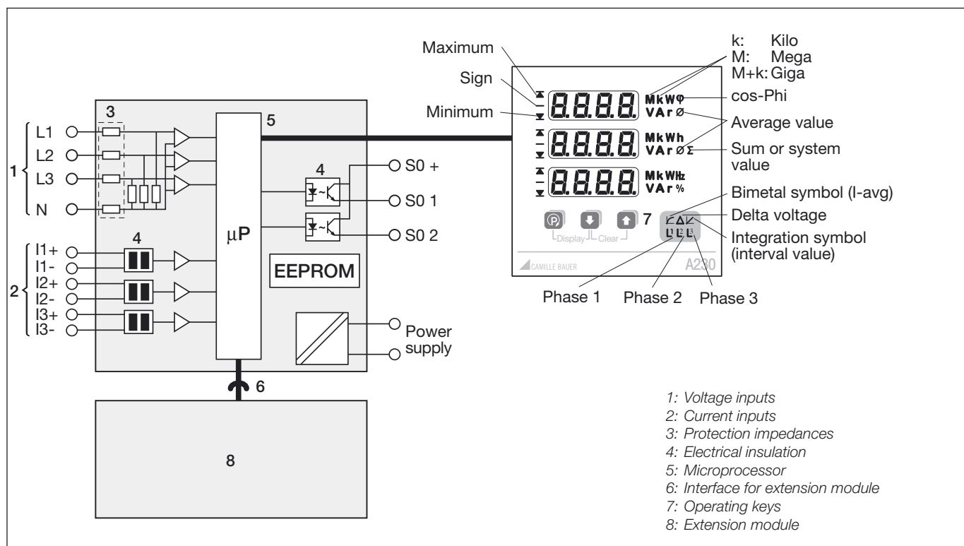
Bild 1. Blockschema
